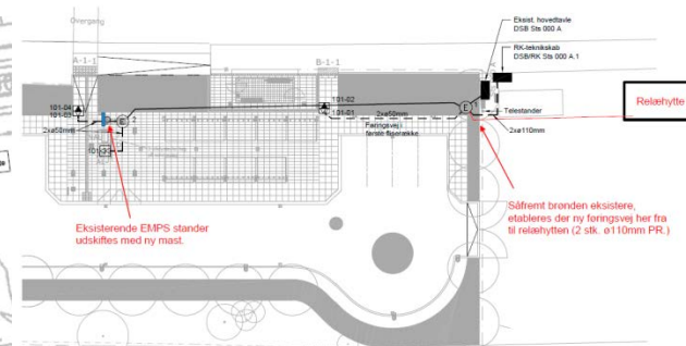
Figur 2 – Plantegning af placeringer og føringsveje på stationen
